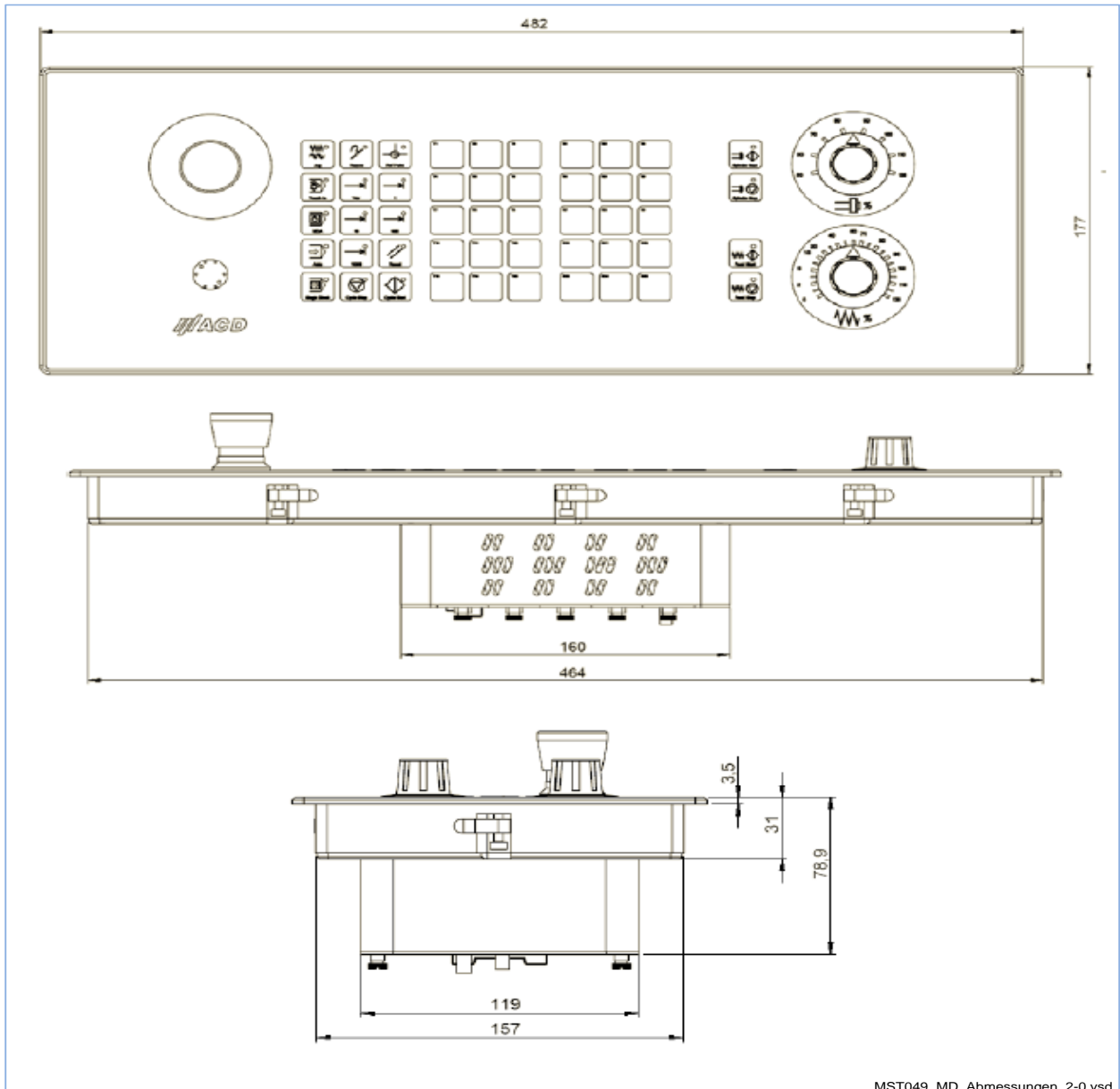
MST049_MD_Abmessungen_2-0.vsd
